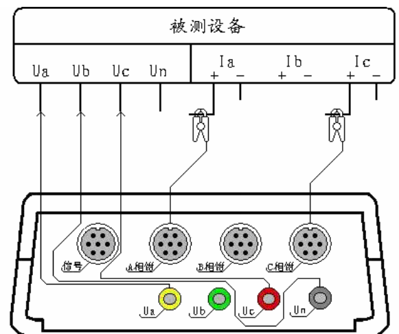
三相三线制设备测试接线图
